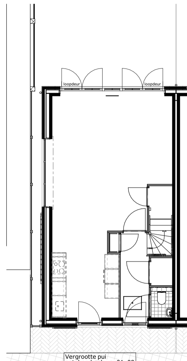
Vergrootte pui getekend: bwnr 01, 09 gespiegeld: bwnr 02, 10
