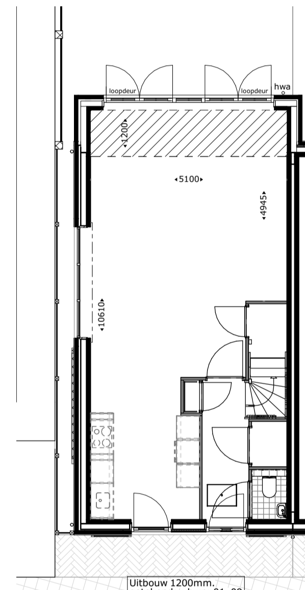
Uitbouw 1200mm. getekend: bwnr 01, 09 gespiegeld: bwnr 02
