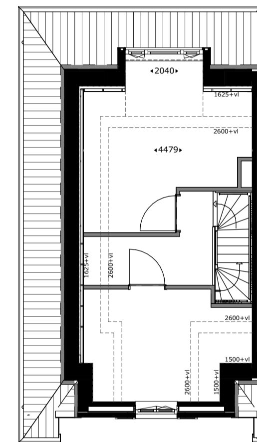
Dakkapel achtergevel getekend: bwnr 01 gespiegeld: bwnr 10
