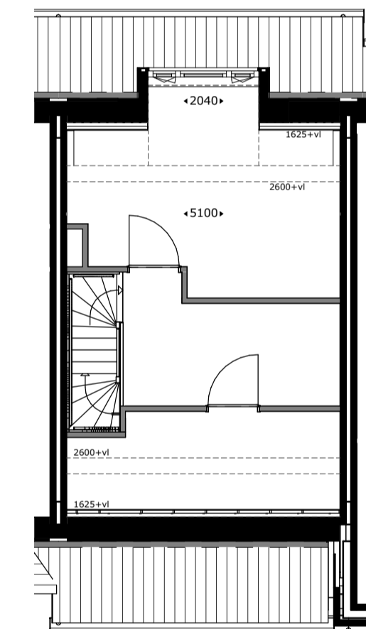
Dakkapel achtergevel getekend: bwnr 02 gespiegeld: bwnr 09
