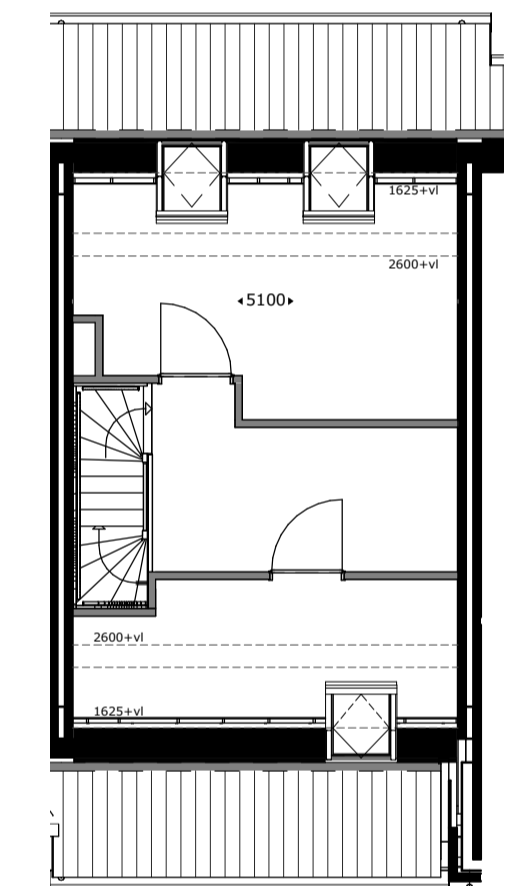
Dakraam voorgevel (vergunningplichtig) getekend: bwnr 02 gespiegeld: bwnr 09
