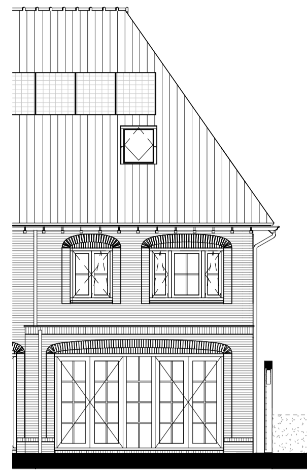
Uitbouw 1200mm. getekend: bwnr 01, 09 gespiegeld: bwnr 02
