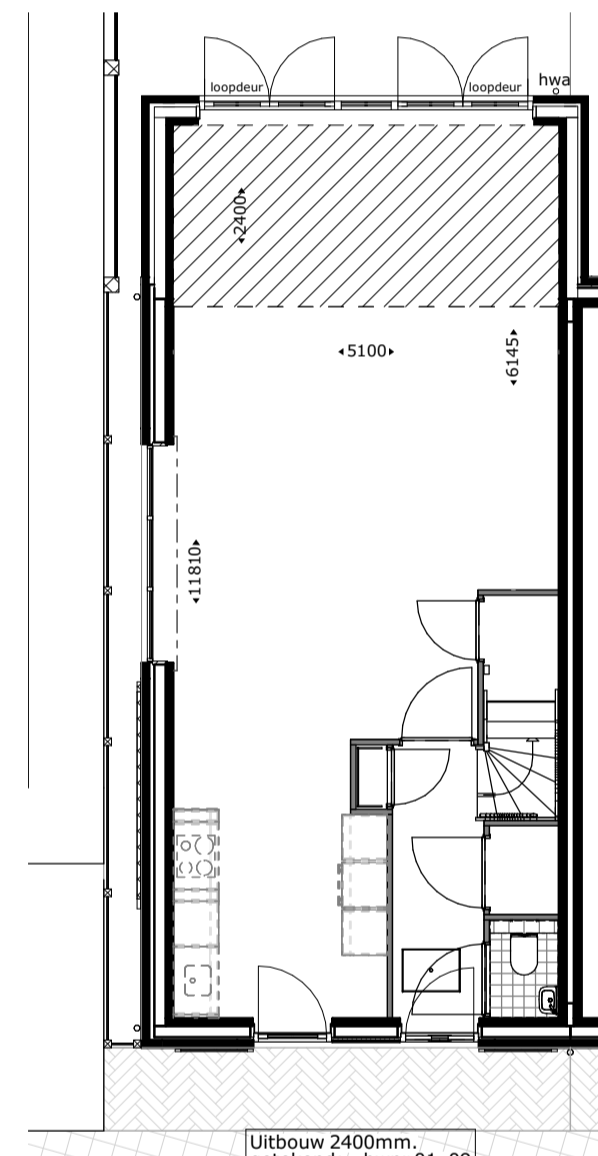
Uitbouw 2400mm. getekend: bwnr 01, 09 gespiegeld: bwnr 02
