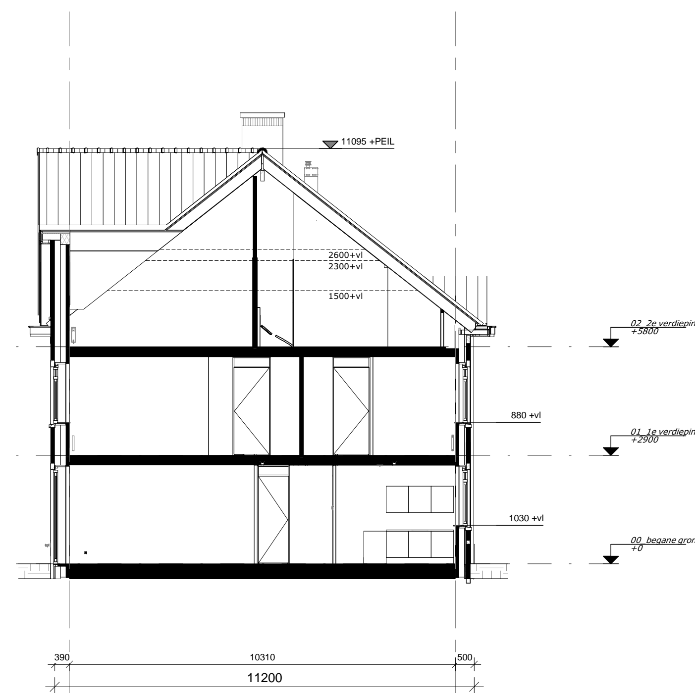
Doorsnede C
