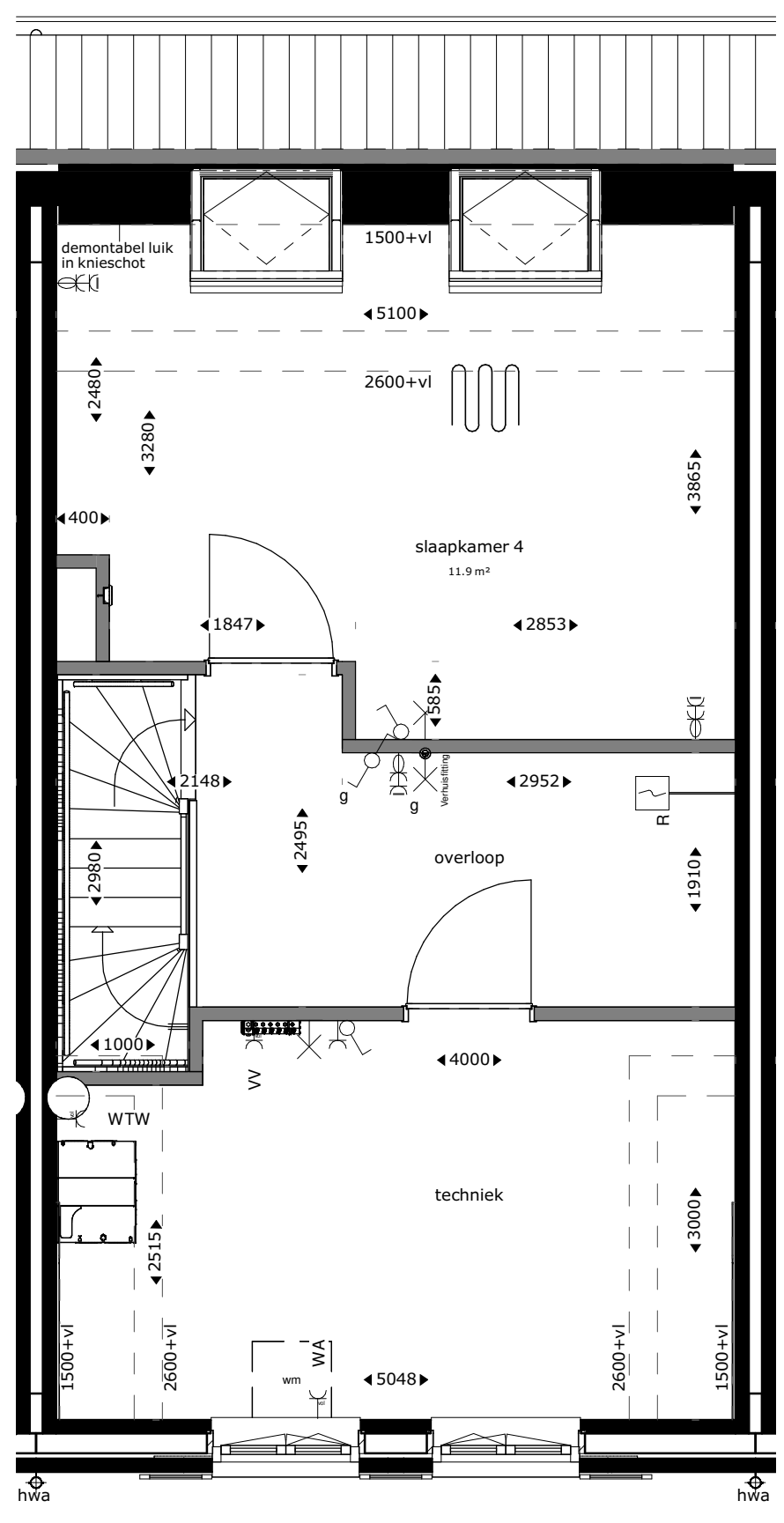
tweede verdieping
