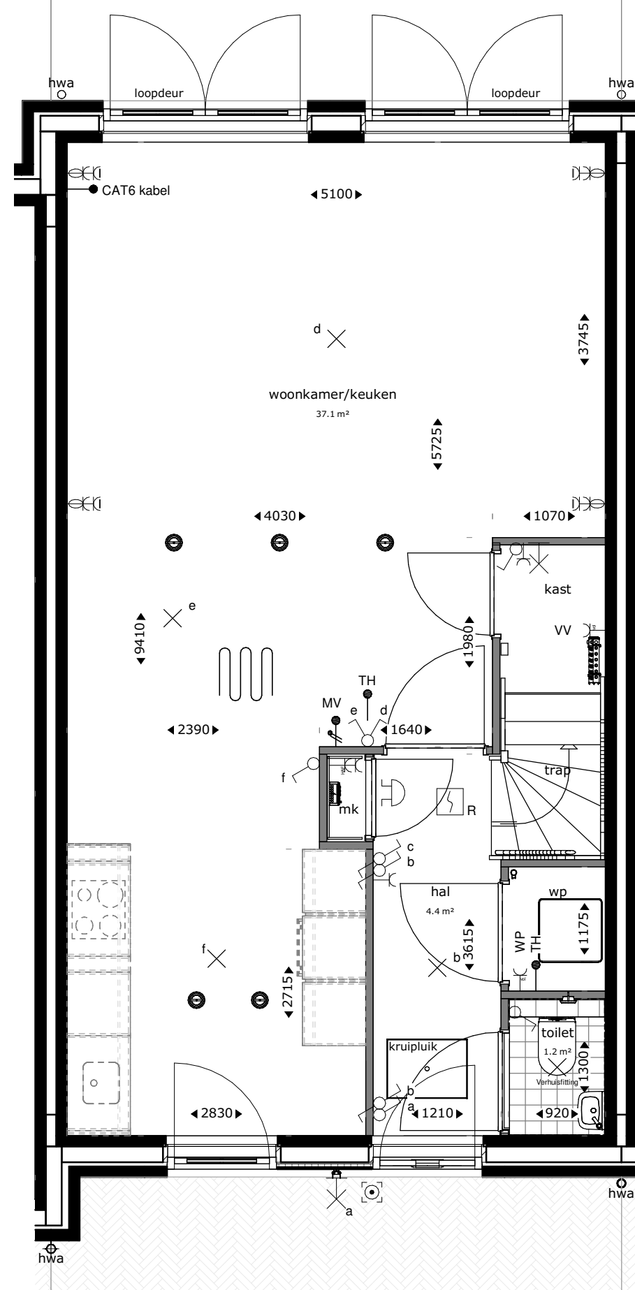
begane grond
