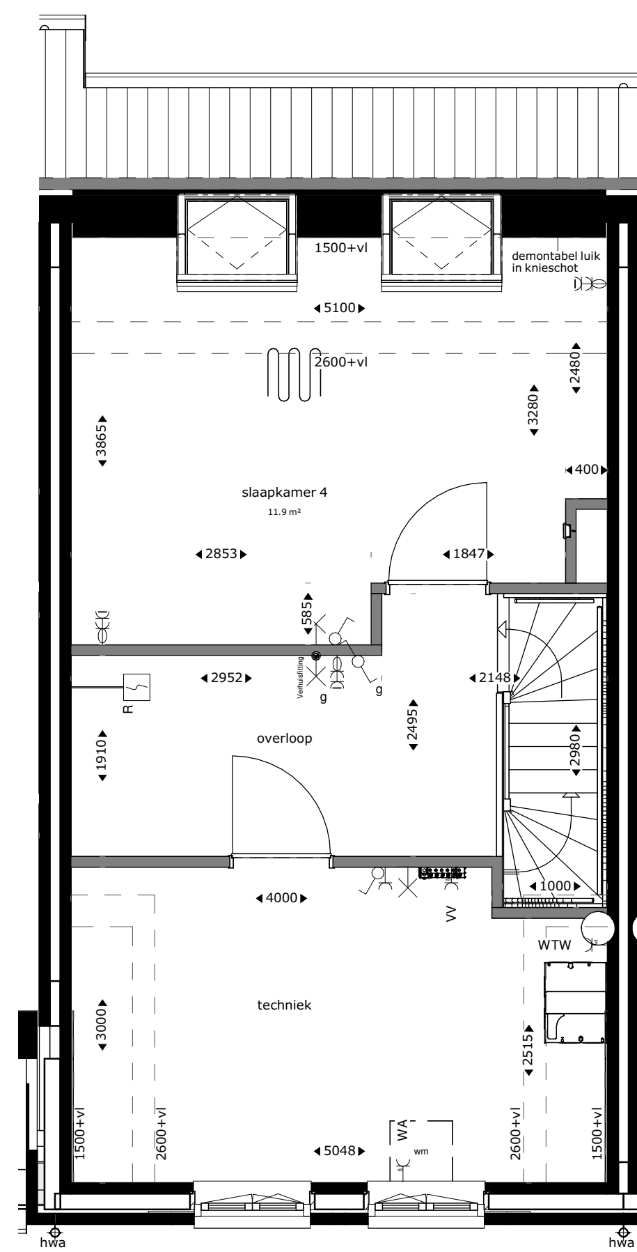
tweede verdieping
