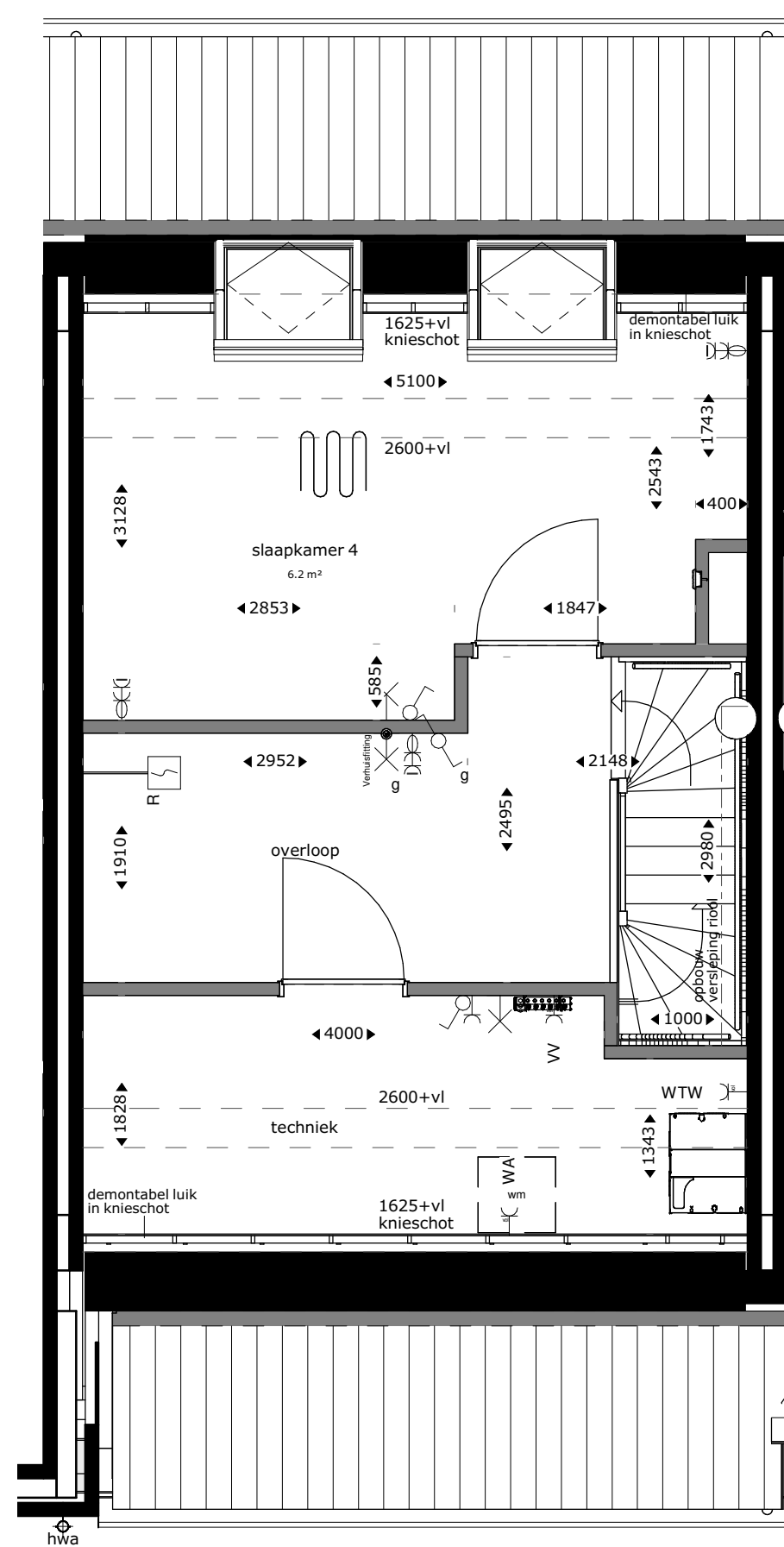
tweede verdieping
