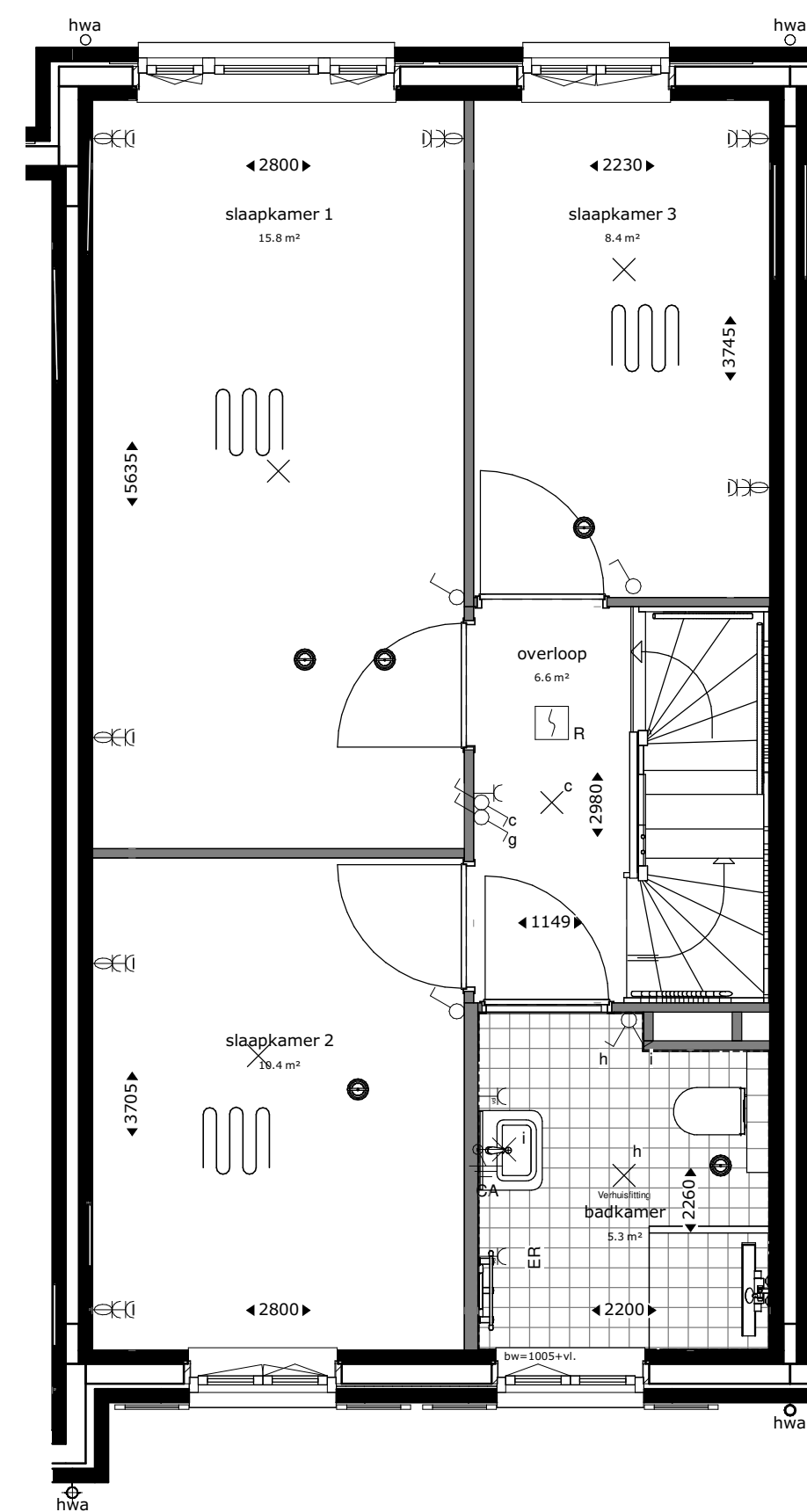
eerste verdieping
