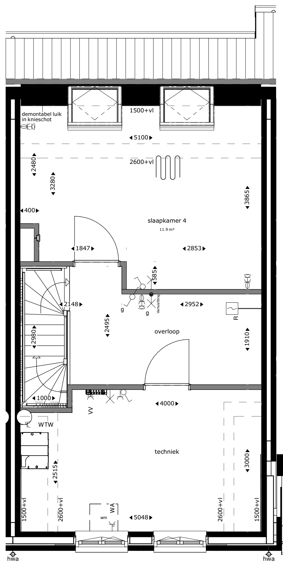
tweede verdieping
