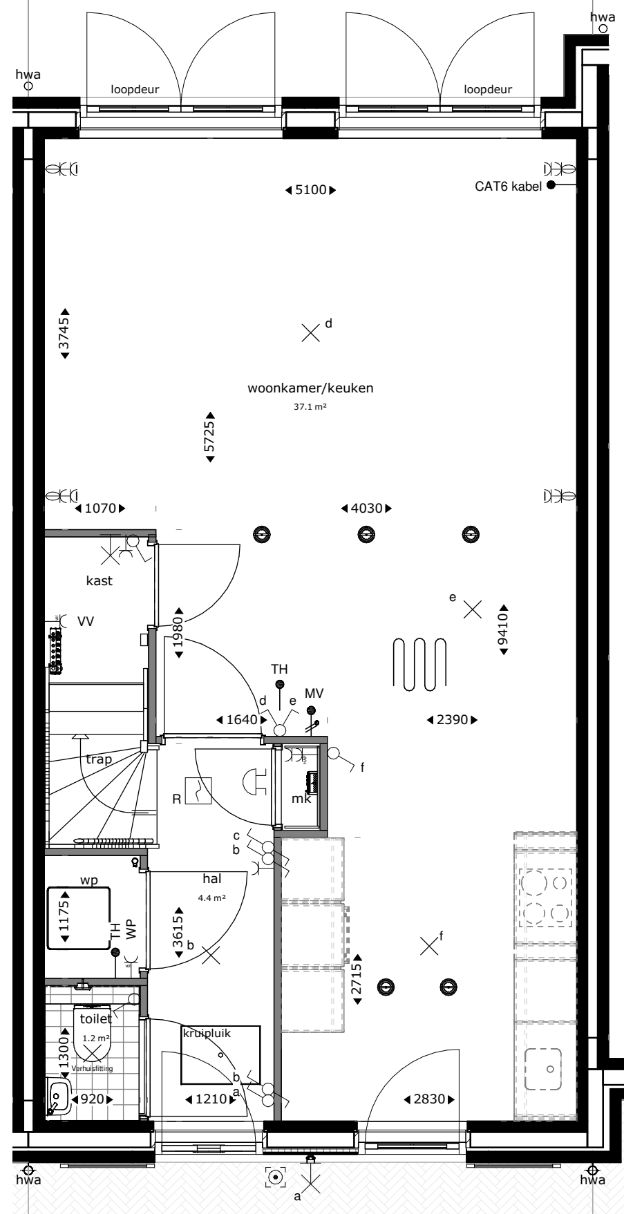
begane grond
