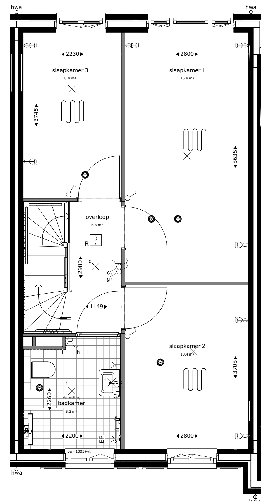
eerste verdieping
