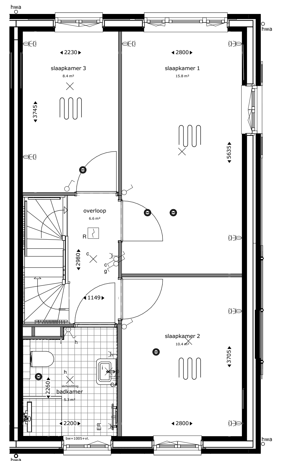
eerste verdieping
