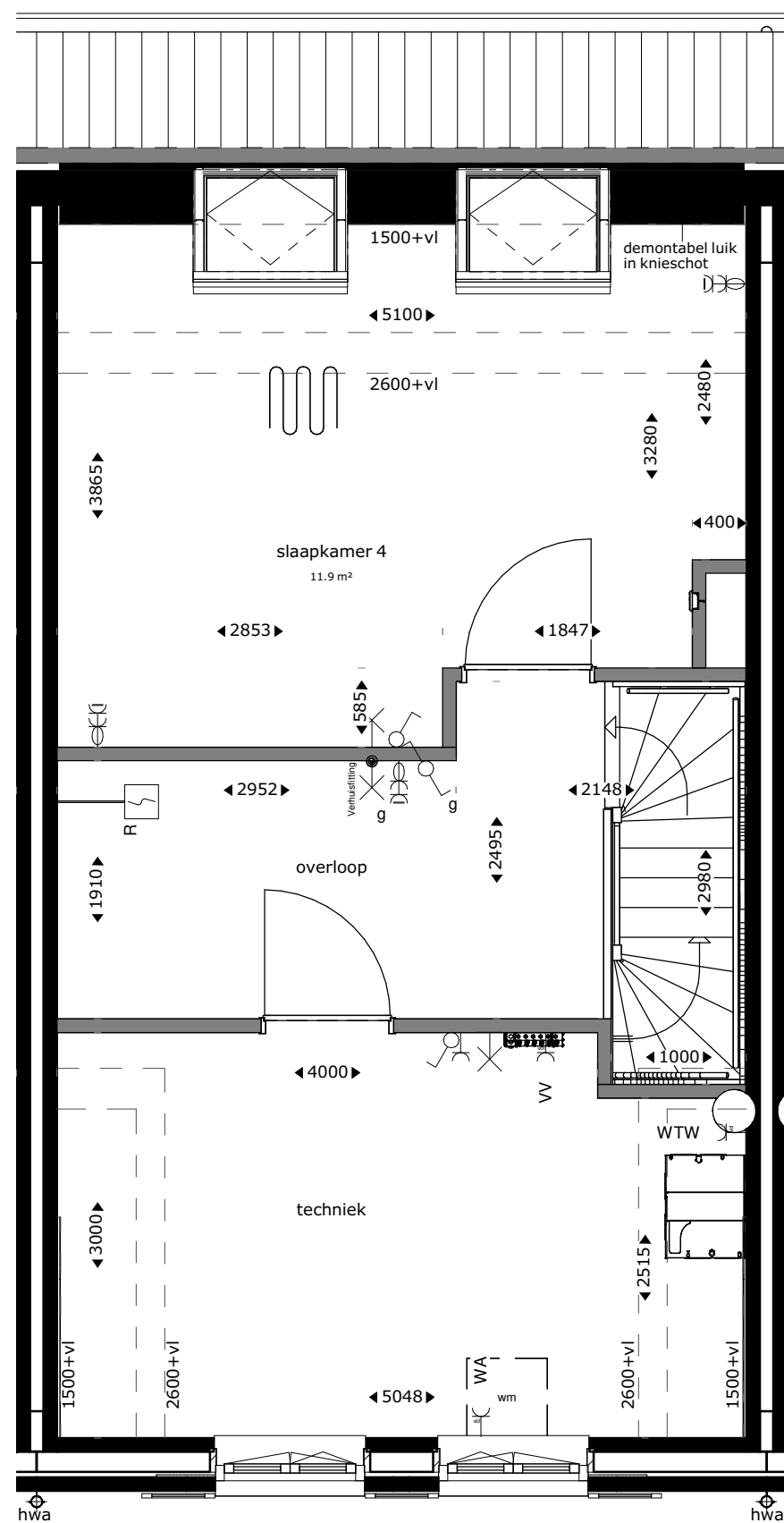
tweede verdieping
